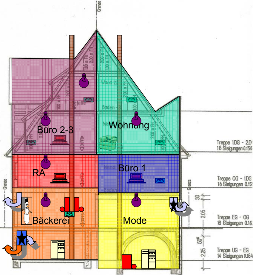
Schnitt A - A M 1/100
