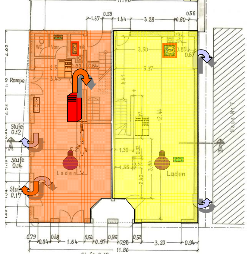
Grundriss Erdgeschoss M 1/100
